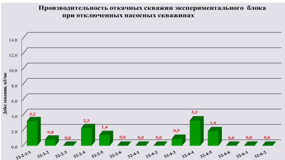
Рисунок 2 Производительность откачных скважин экспериментального блока при отключенных насосных скважинах
